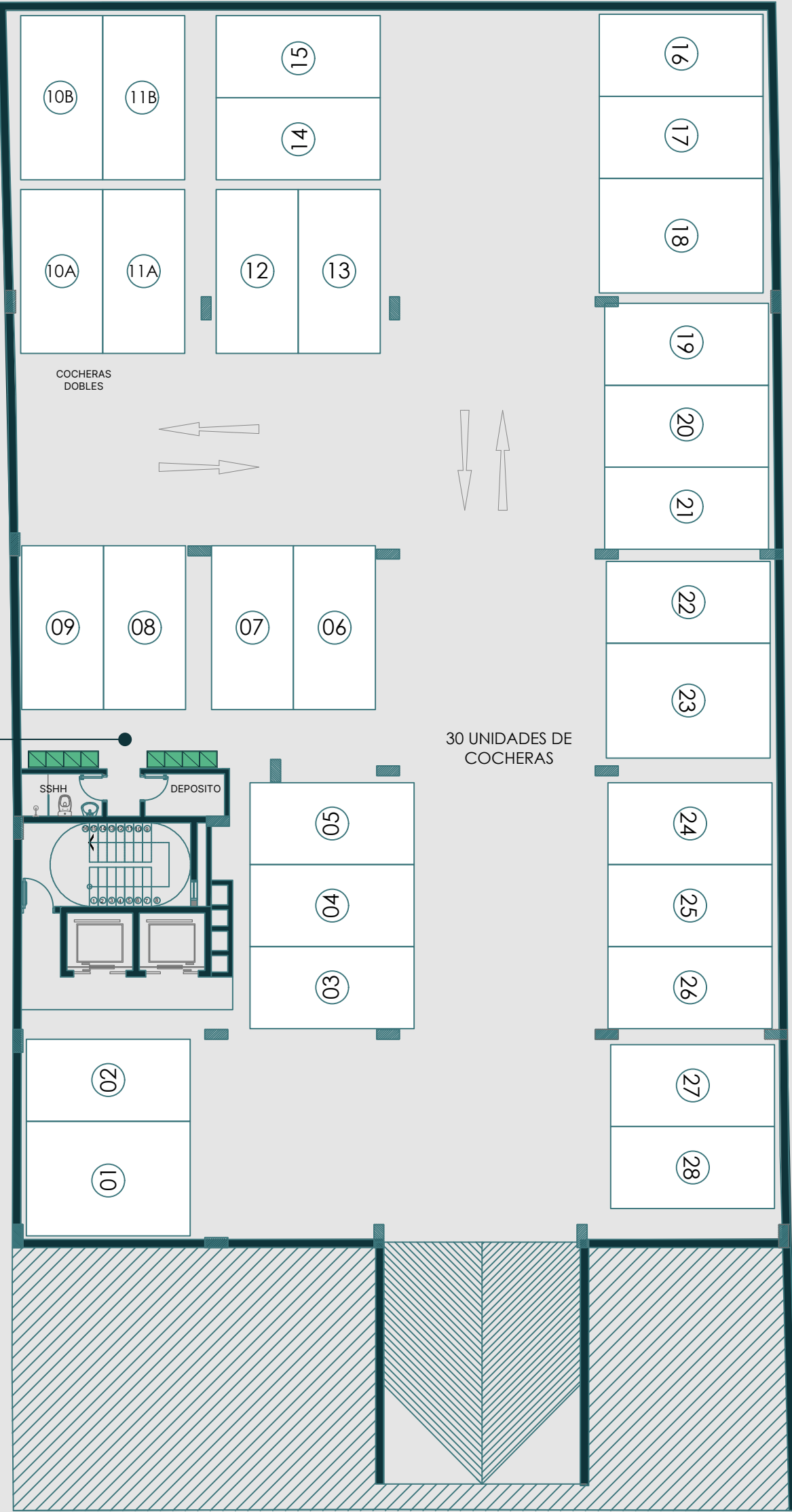
PLANTA SEMI SUBSUELO 30 Cocheras
